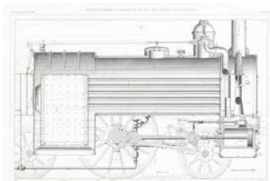
Locomotive la Gironde dans Publication industrielle des machines, outils et appareils , Paris, E. Armengaud, 1857 à 1890 © Écomusée Creusot Montceau.
